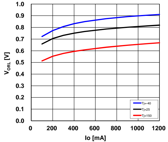
I_o vs. V_{ORL} V_{MM}=24V
