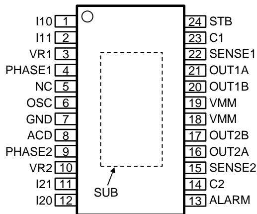
HTSSOP24-P1
