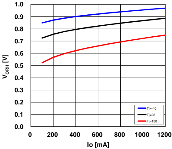
I_o vs. V_{ORH} V_{MM}=24V
