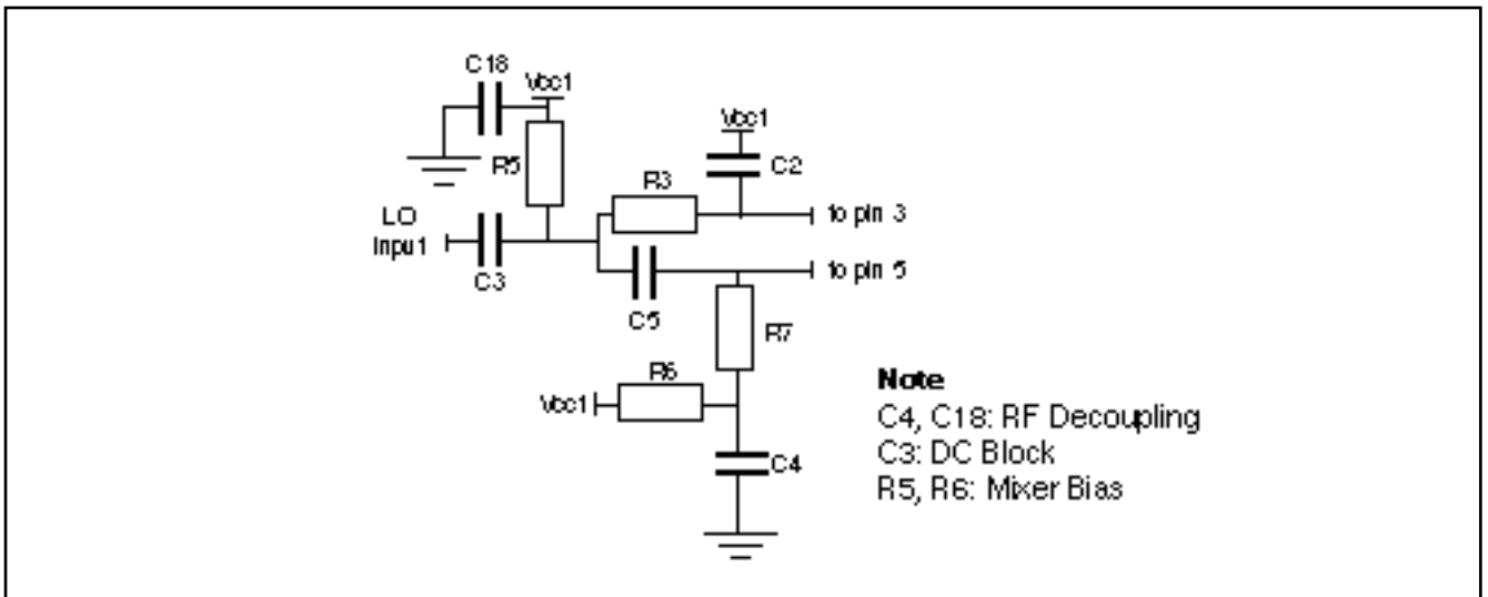
Fig.5 LO Network
