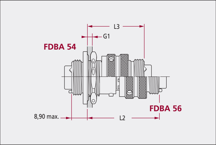
Jam nut receptacle / Collettte ronde
