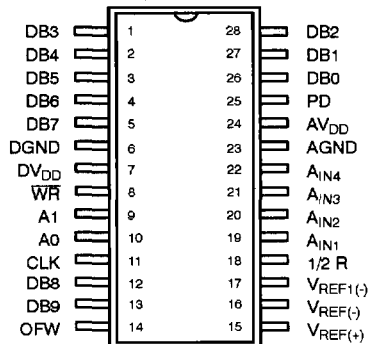
28 Pin SOIC (Jedec, 0.300") 28 Pin SSOP
