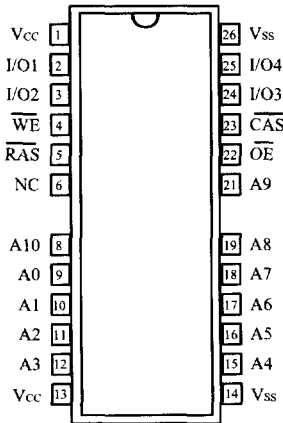
24(26)SOJ
