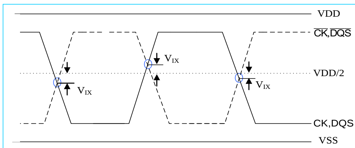
Fig. 62: V_{IX} Definition
