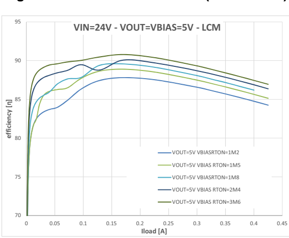
Figure 34. VIN 24 V - VOUT 5 V (linear scale)
