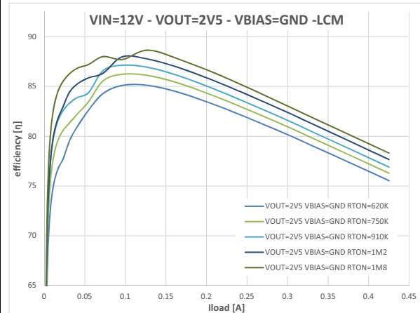
Figure 40. VIN 12 V - VOUT 2.5 V (linear scale)
