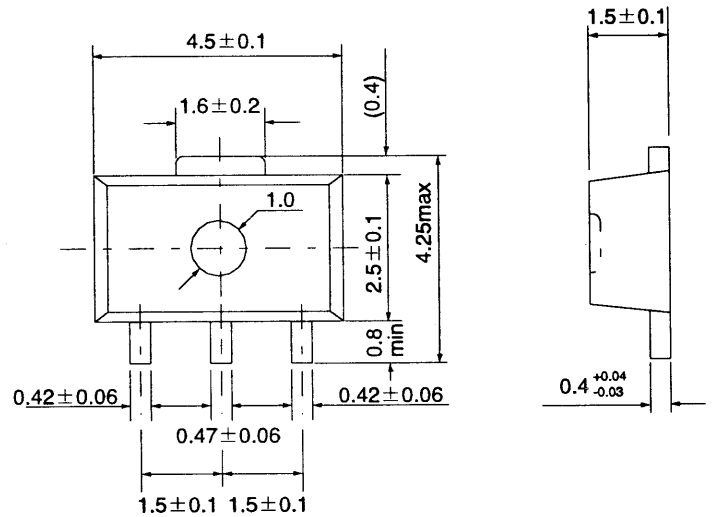
SOT-89
