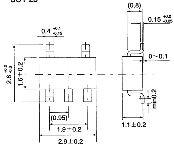
SOT-25
