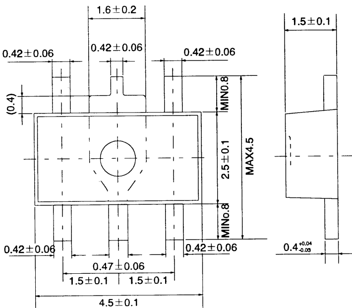
SOT-89-5
