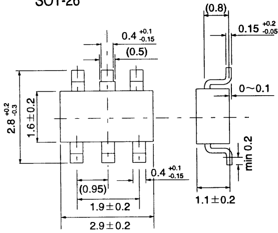
SOT-26
