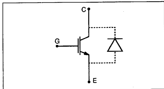
Fig. 2 ITE35X12 circuit
