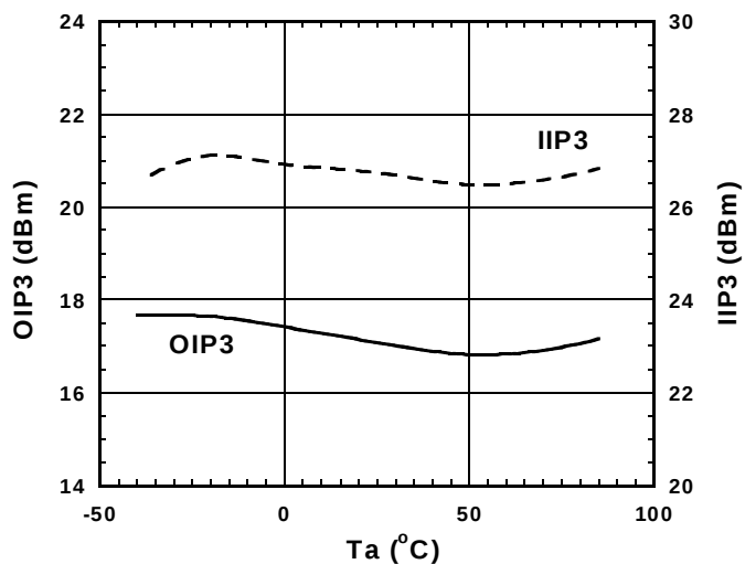
OIP3, IIP3 vs. Ta
