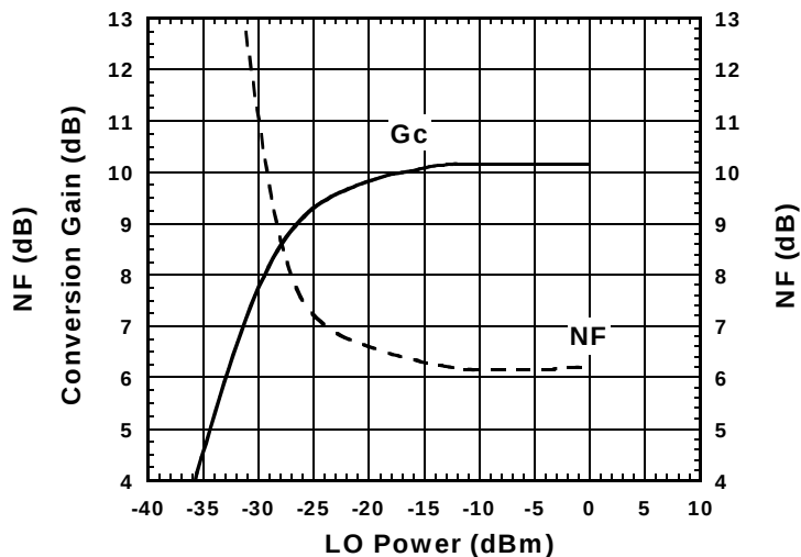
Gc, NF vs. LO Power
