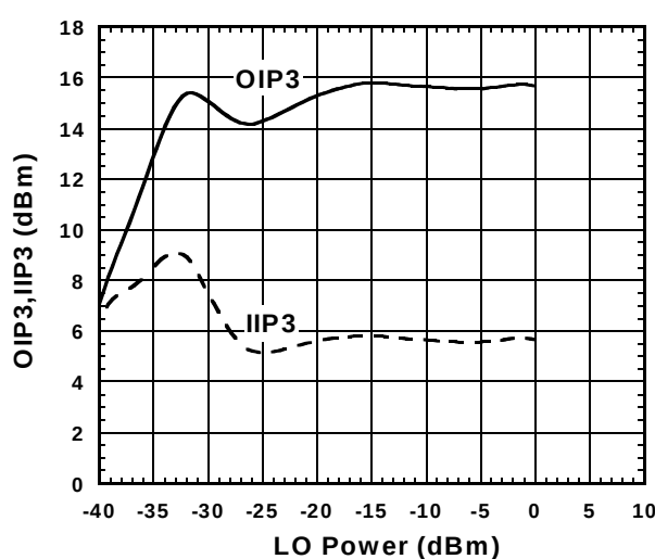
OIP3, IIP3 vs. LO Power
