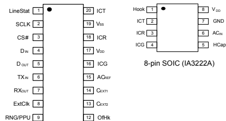
20-pin QSOP (IA3223A)
