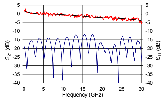
NIR-MX-LN-20: S_{21} & S_{11} Parameter Curves
