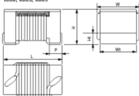
1008, 0805, 0603
