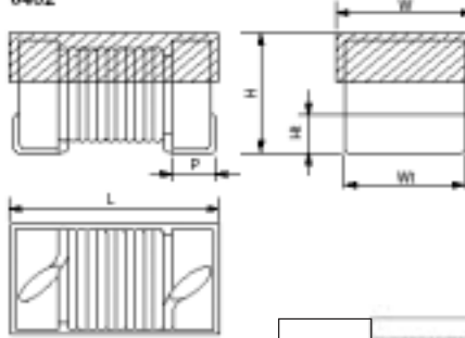
0402
