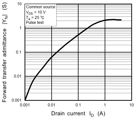
Fig. 7.9 |Y_{fs}| - I_D
