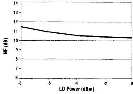
NF vs. LO Power
