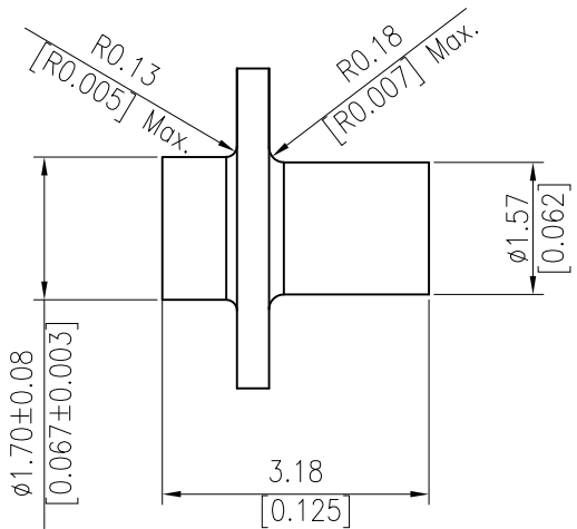
SCE A-A SCALE 1:1
