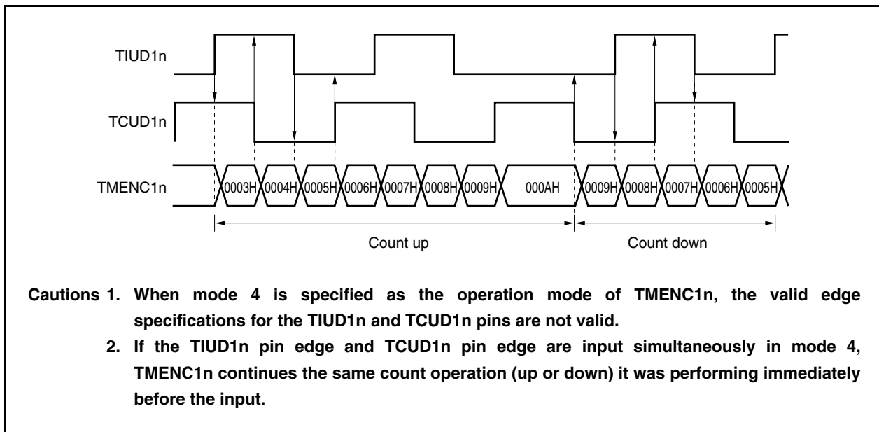
Figure 8-9. Mode 4
