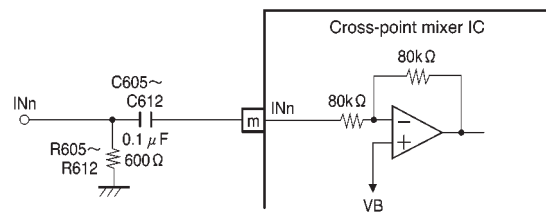
Fig. 6 Input circuit
