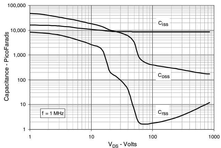
Fig. 12. Capacitance
