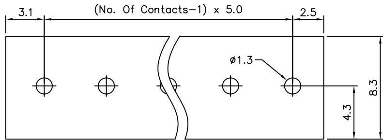
P.C.B Layout
