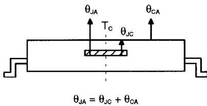
Thermal Resistance — °C/Watt
