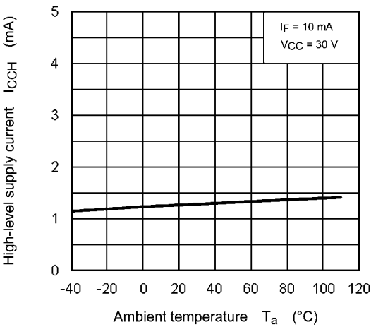
Fig. 13.2.6 I_{CCH} - T_a
