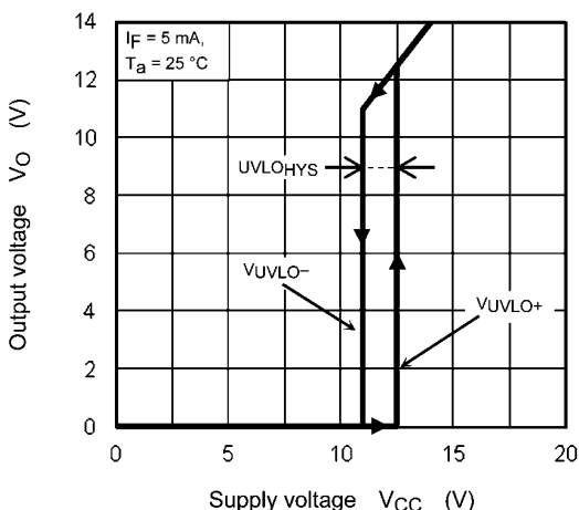
Fig. 13.2.11 V_O(V_{UVLO}) - V_{CC}
