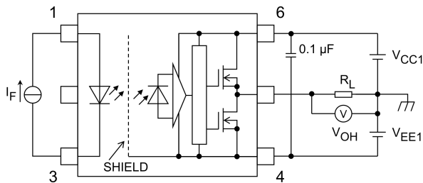
Fig. 13.1.3 V_{OH} Test Circuit
