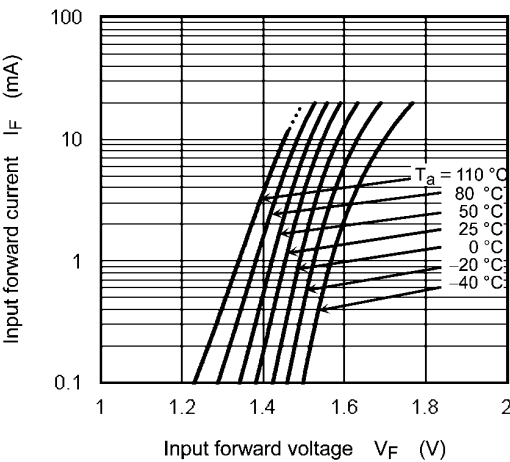
Fig. 13.2.1 I_F - V_F
