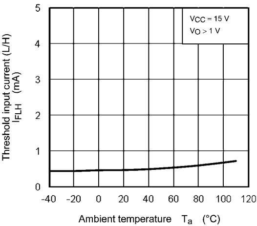
Fig. 13.2.4 I_{FLH} - T_a
