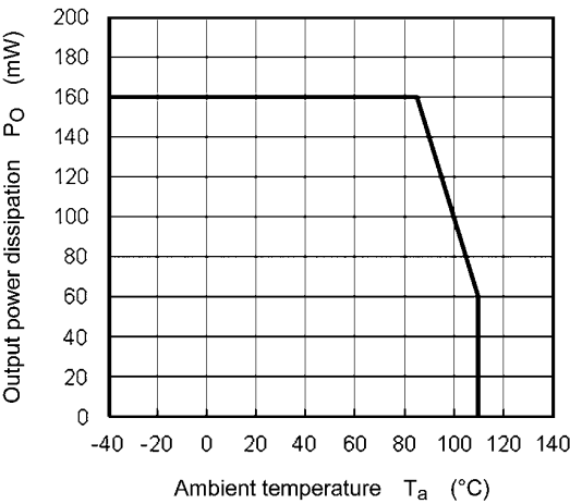
Fig. 13.2.3 P_O - T_a
