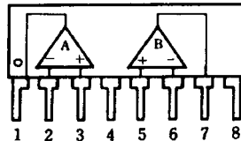
NJM4565L
