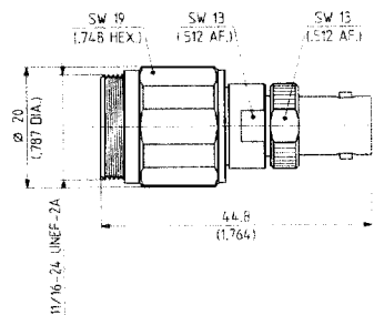
TYPE 33 PC7-BNC-50-1
