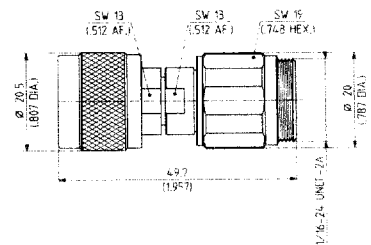
TYPE 32 N-PC7-50-1
