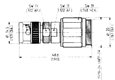
TYPE 32 BNC-PC7-50-1
