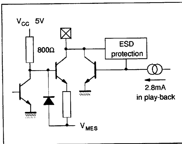
Pin : Iout
