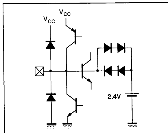
Pin : CAGC
