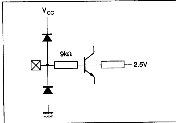
Pin : VREC
