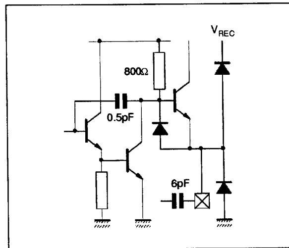
Pin : CAGC
