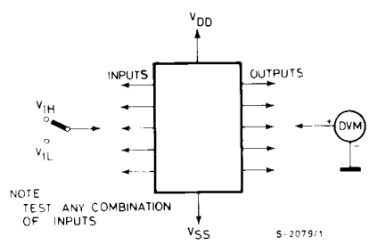
Input voltage
