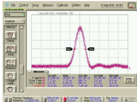
NIR-MX800-LN-20: 30 ps Square Pulse
