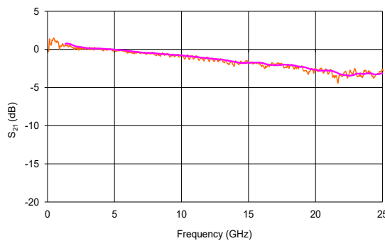
NIR-MX800-LN-20: 30 ps Square Pulse
