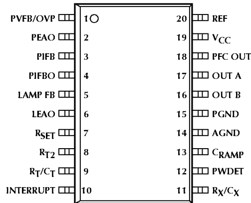
ML4835 20-Pin SOIC (S20) 20-Pin DIP (P20)
