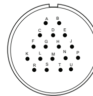
36A16 18 #12 (B,C,V,J,K,M,N, R, T-Iron; A,D-F,H,L P,S,U-Constantan)
