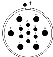
40A33 7 #8(G-N) 6 #4(A-F)
