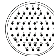
36A66 52 #16(A-c,h-AK) 4 #12(d,e,f,g)
