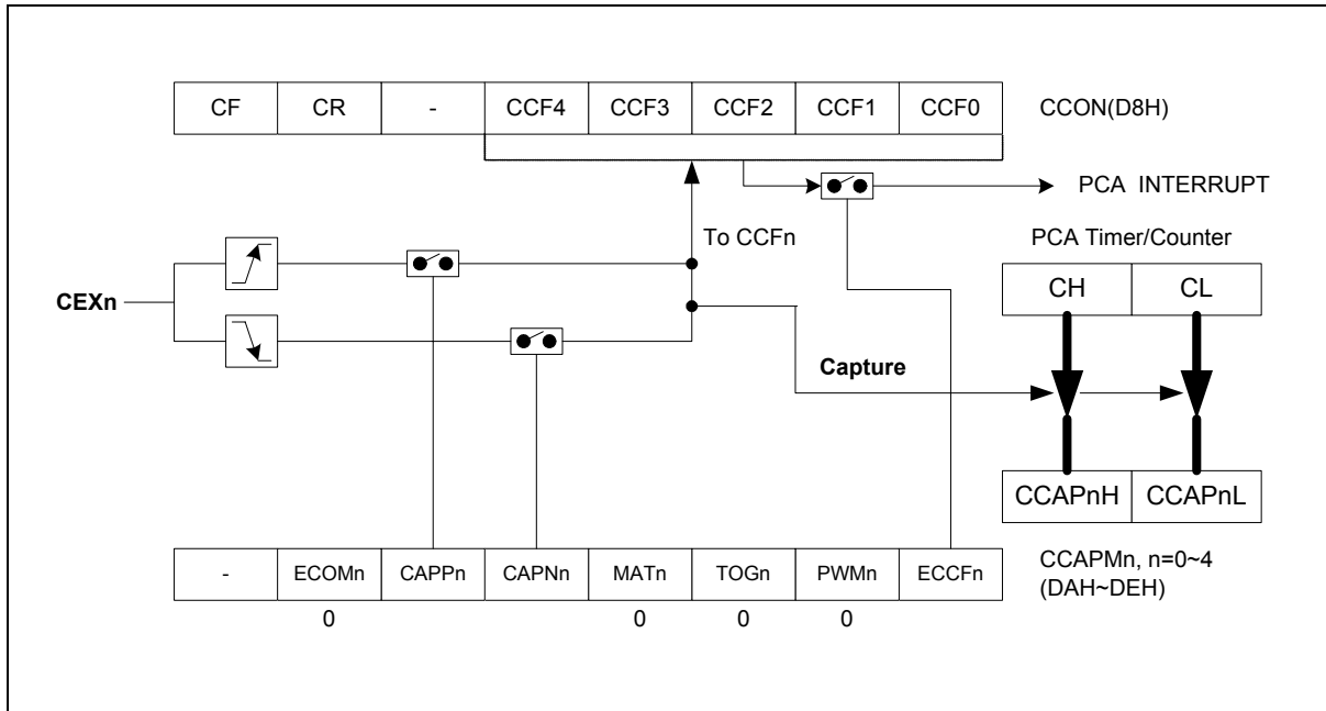
PCA Capture Mode
