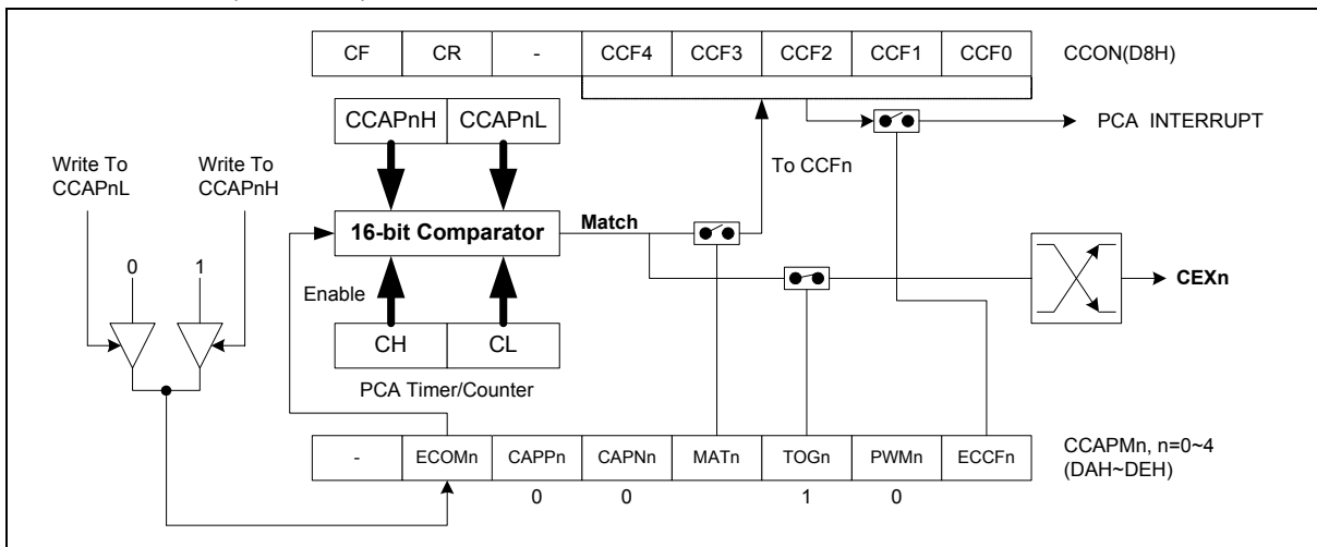
PCA High Speed Output Mode
