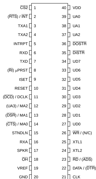
600-Mil 40-Pin DIP 73K222AU-IP
