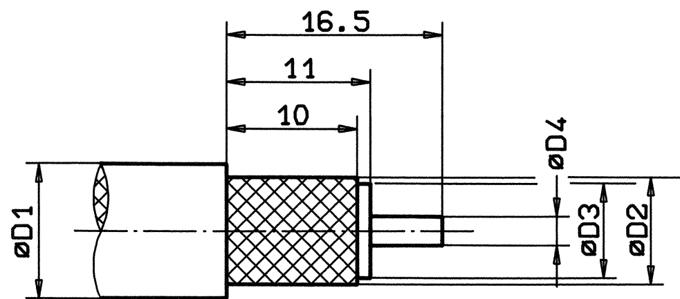
KABELZUSCHNITT M2.5:1
