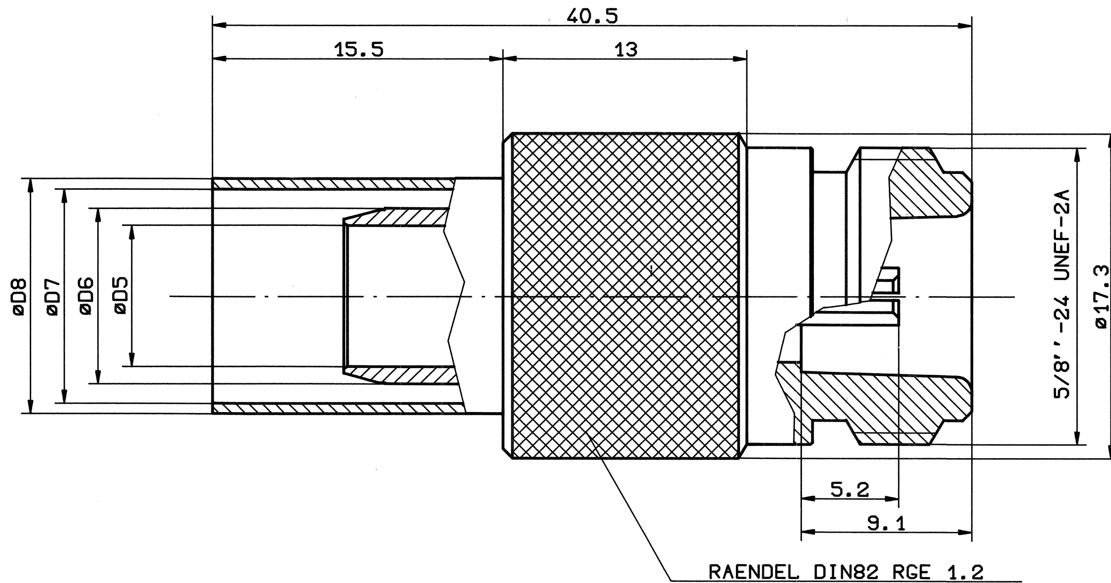
KABELZUSCHNITT M2.5:1
