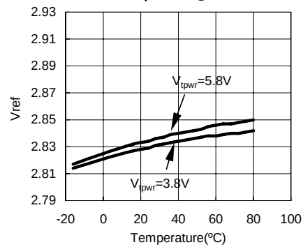
Vref - Temperature@Ivref=0mA
