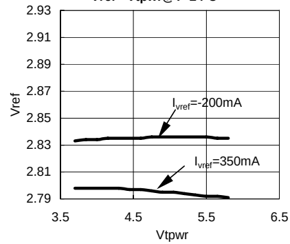
Vref - Vtpwr@T=24°C
