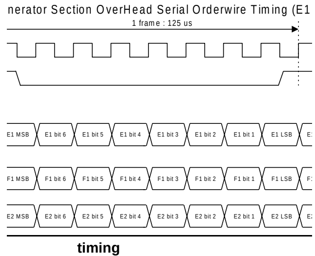
Figure 21: Transmit orderwire E1, E2 and F1
