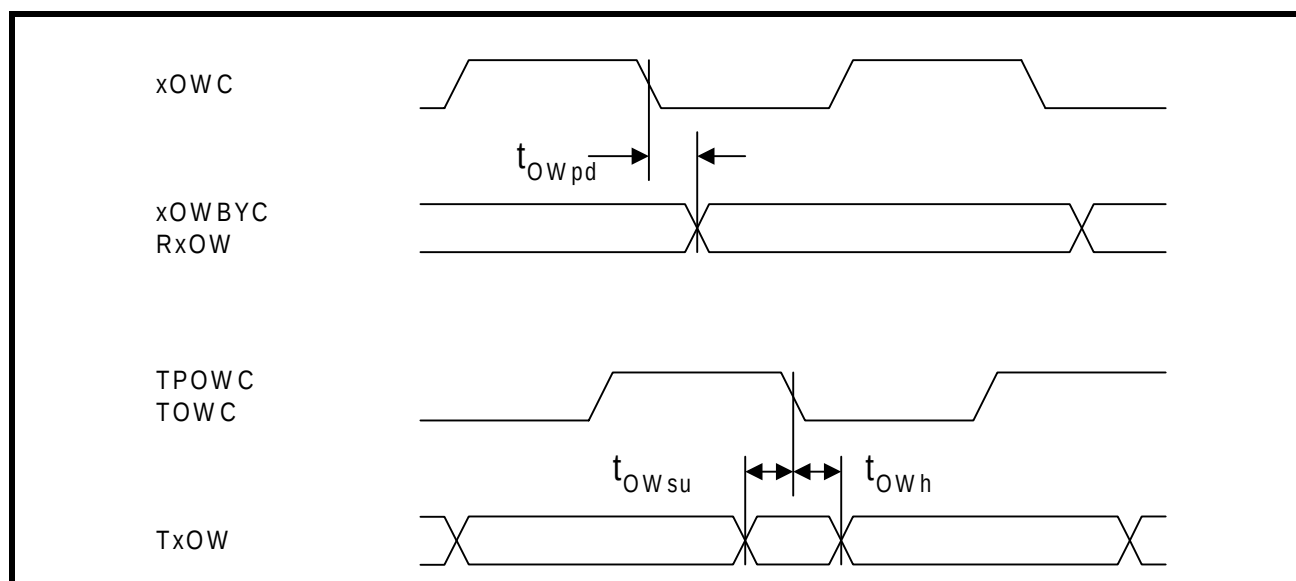
Figure 44: Orderwire E1, F1 &amp; E2, F2 &amp; F3 Timing
