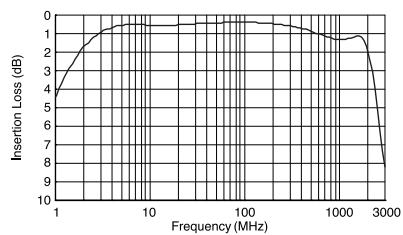
3) #617DB-1655=P3 50Ω:50Ω
