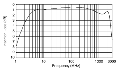
4) #617DB-1724=P3 50Ω:50Ω
