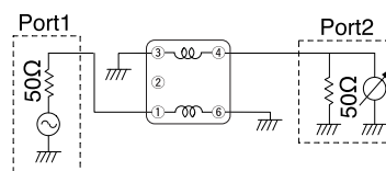
2) #617DB-1654=P3 50Ω:50Ω
