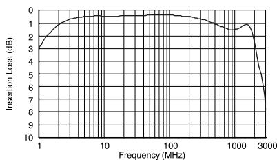
4) #617DB-1724=P3 50Ω:50Ω
