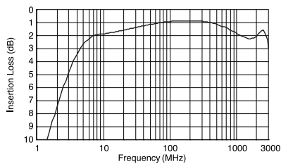
3) #617DB-1655=P3 50Ω:50Ω
