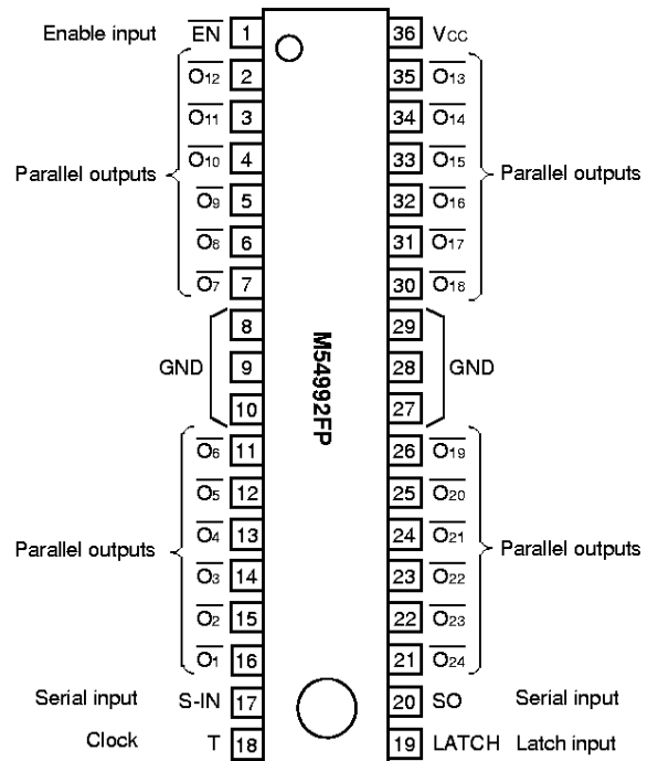
Outline 36P2R-A
