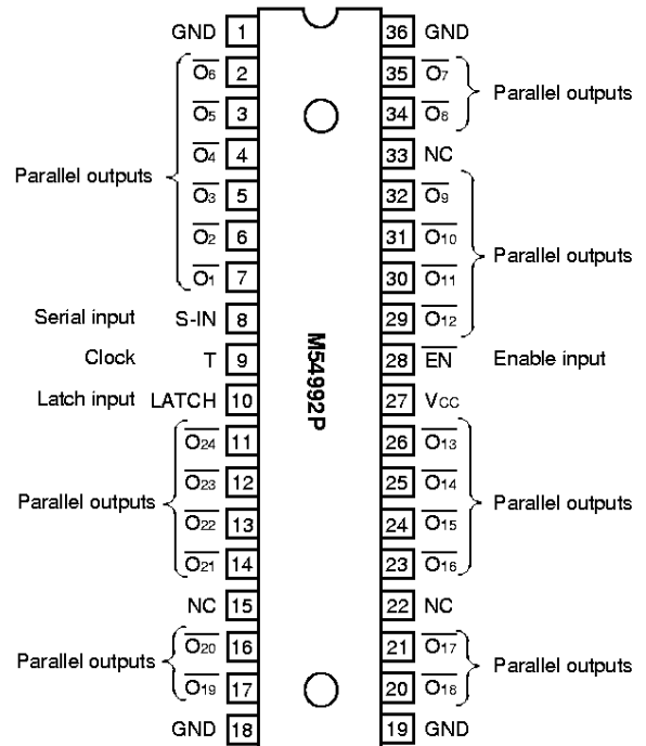
Outline 36P4E
