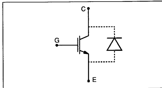
Fig. 2 ITE15X12 circuit
