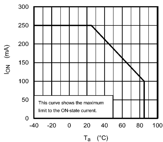
Fig. 14.2 I_{ON} - T_a
