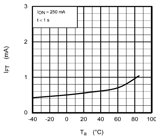
Fig. 14.6 I_{FT} - T_a
