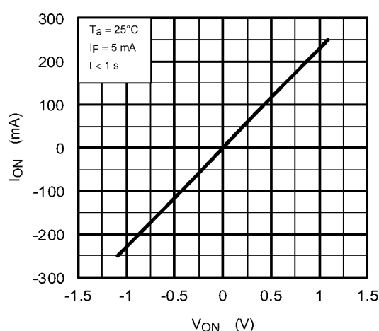
Fig. 14.4 I_{ON} - V_{ON}
