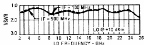
I-Port VSWR
