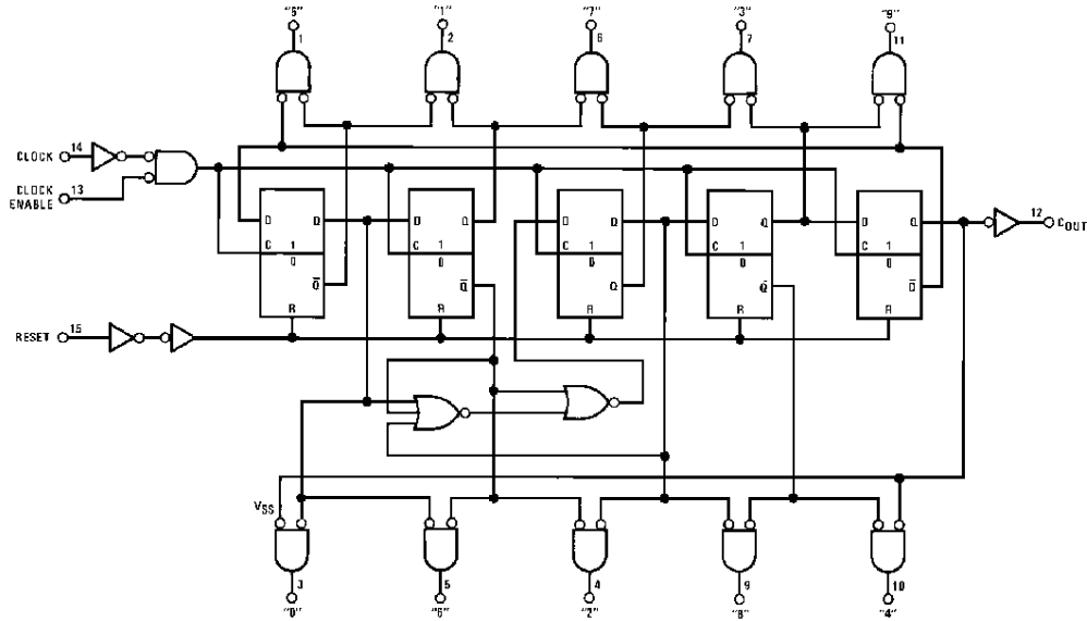
CD4017B
