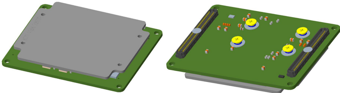
Figure 1: K26 SOM
