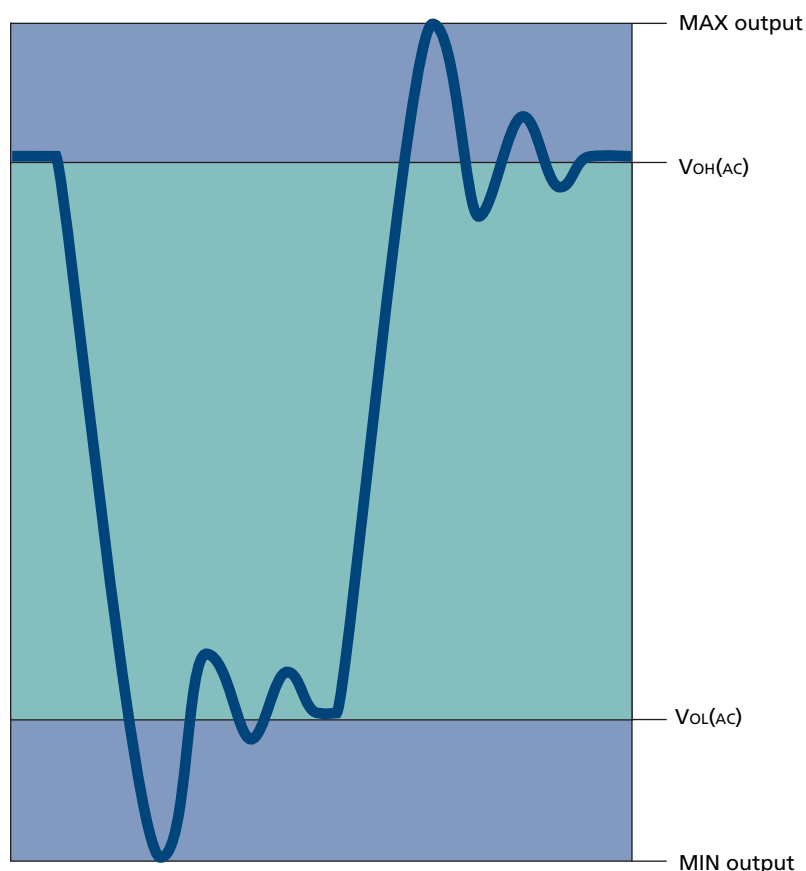
Figure 27: DQ Output Signal
