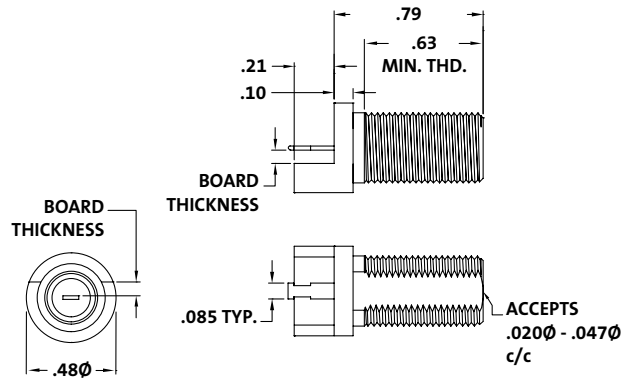
PCB Edge Mount
