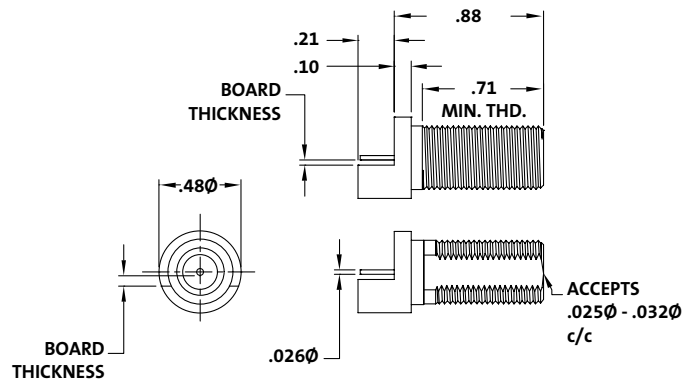
2 GHz Edge Mount
