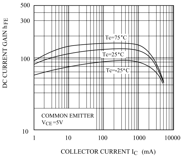
h_{FE} - I_C
