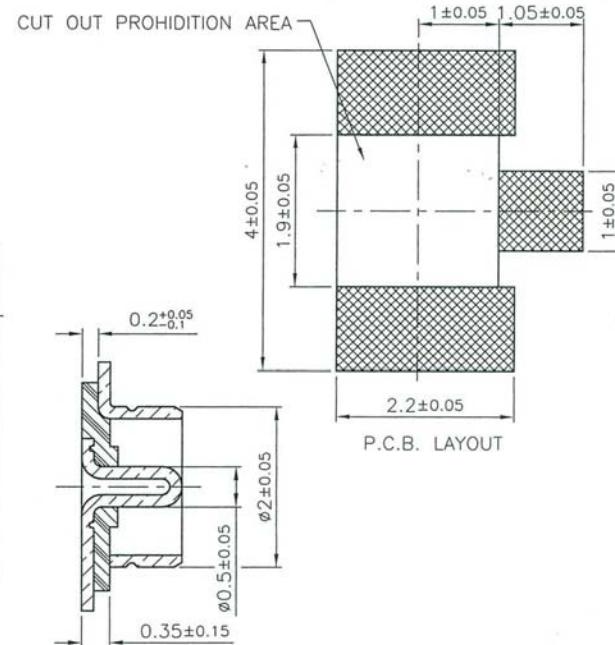
A-A' SECTION (A-A' 剖面)
