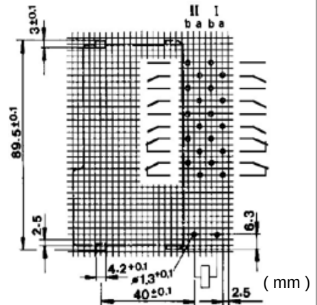
6NO/4NC PACKAGE
