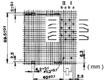
3NO/3NC PACKAGE
