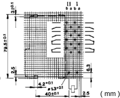
4NO/4NC PACKAGE
