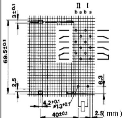
4NO/2NC PACKAGE
