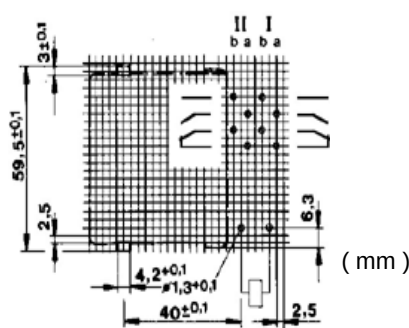
2NO/2NC PACKAGE
