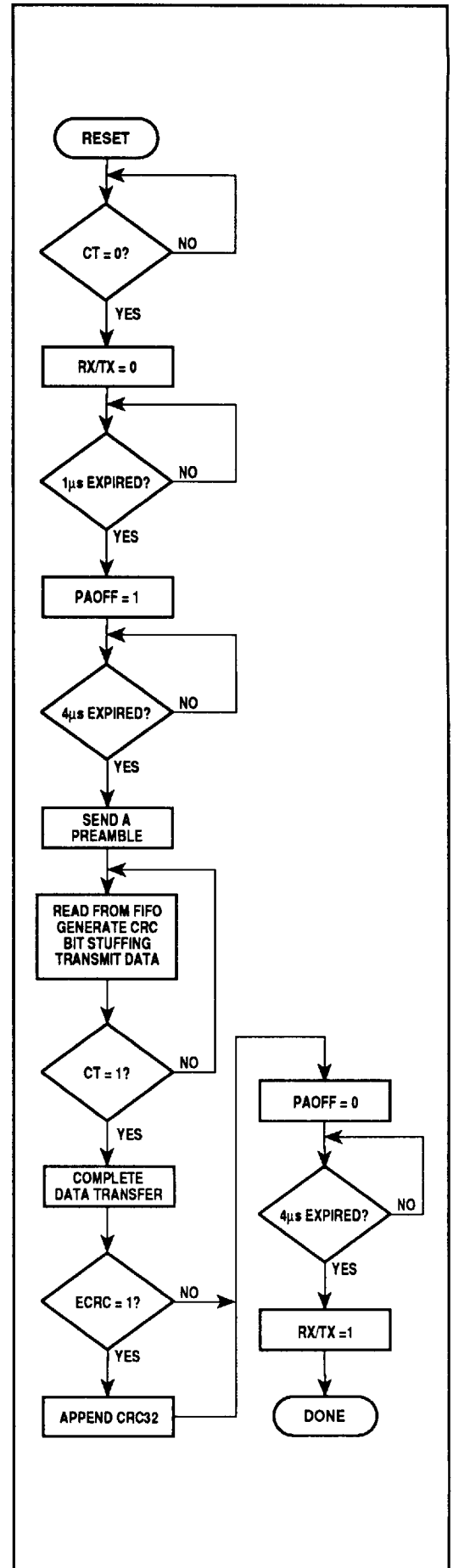
Fig. 13 Data transmit
