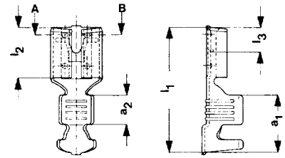
Schnitt A-B
