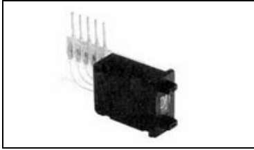
PICOD137ALULS (1571506-1)
