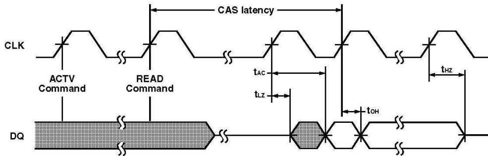
Figure 3: Output Parameters
